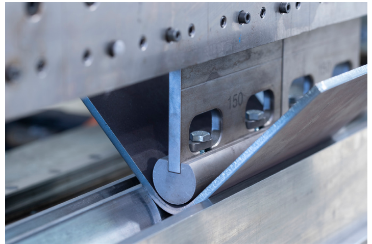
Abbildung 2: Abkantpresse mit 90°-V-Gesenk.
