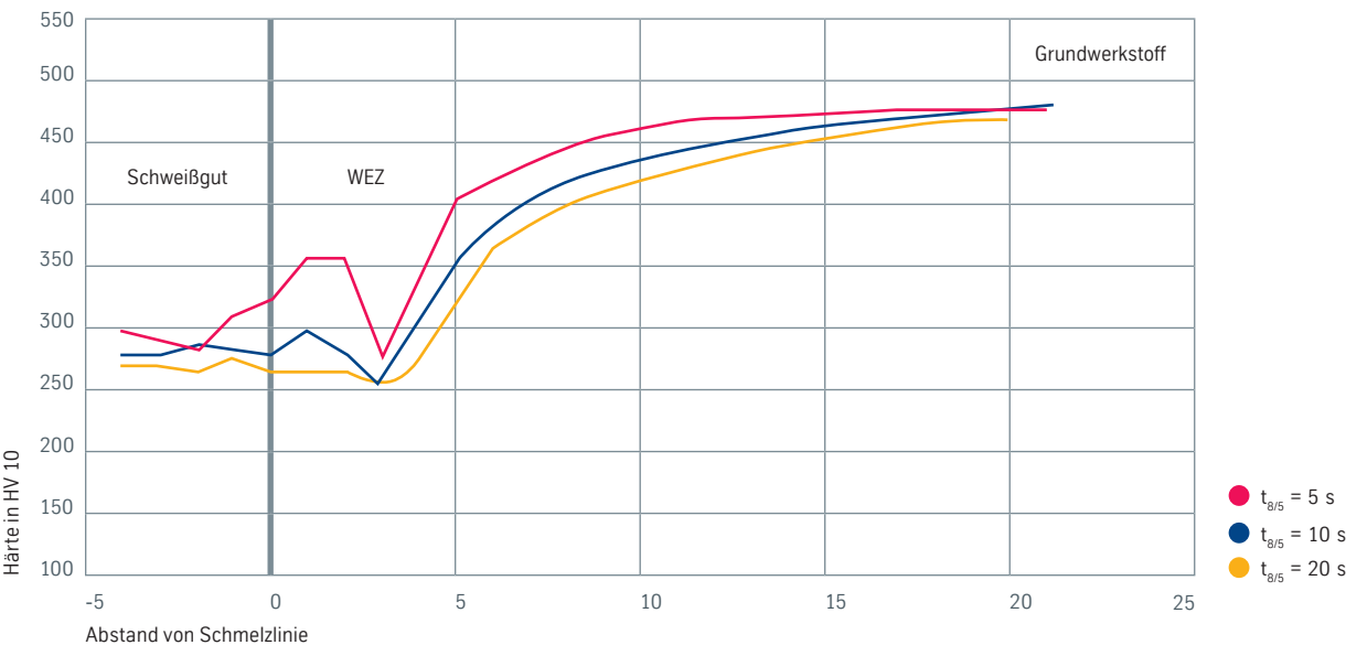
Abbildung 6: Typische Härteverläufe für verschiedene Abkühlzeiten t_{8/5} für perdur® 450
