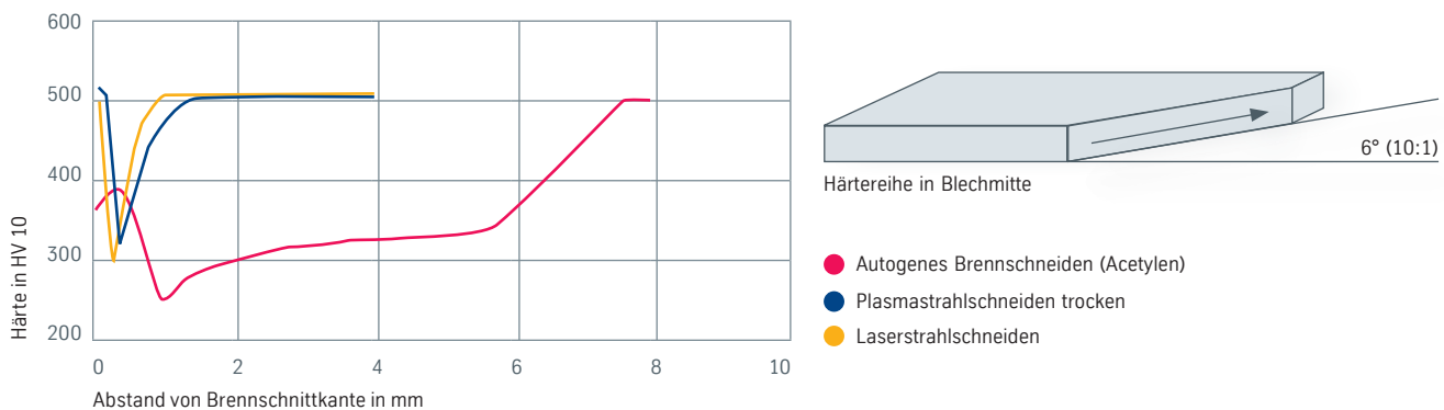
Abbildung 4: Thermisches Schneiden von perdur® 450 (Härteverlauf in der Wärmeeinflusszone)
