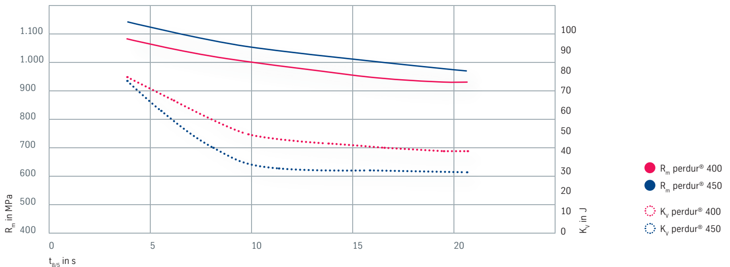
Abbildung 7: Typischer Verlauf der Kerbschlagarbeit und Zugfestigkeit in Abhängigkeit der Abkühlzeit t_{8/5} , Blechdicke 6 mm
