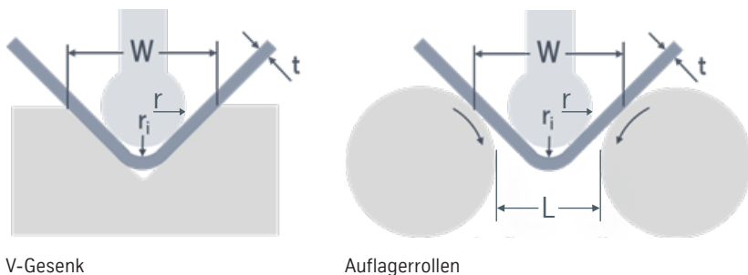
V-Gesenk
