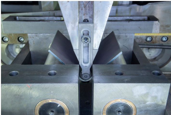
Abbildung 1: Biegevorrichtung mit Auflagerrollen.
