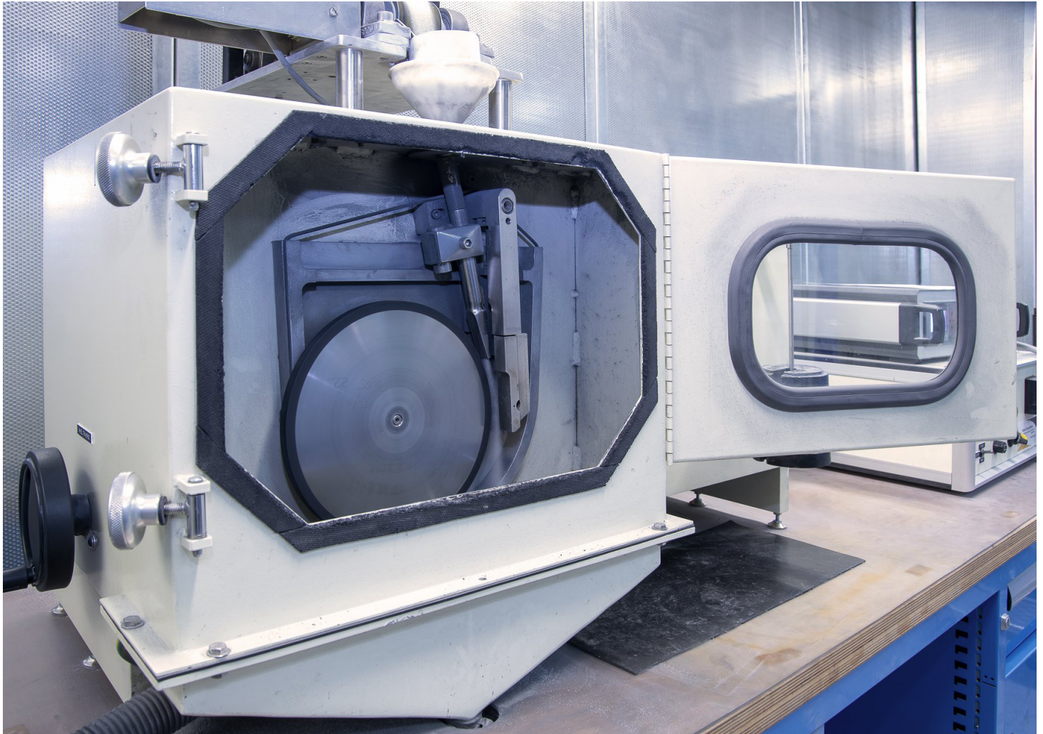
Bei thyssenkrupp Steel betriebener Verschleißprüfstand.
