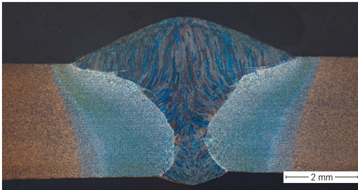
Abbildung 5: MSG-Schweißung an perdur® 450, Blechdicke 6 mm
