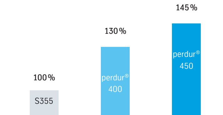
Abbildung 8: Relative Lebensdauer von perdur® versus S355MC
